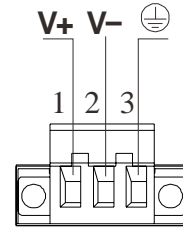
图1 电源输入接口
