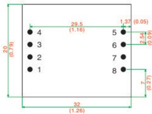
正视图
